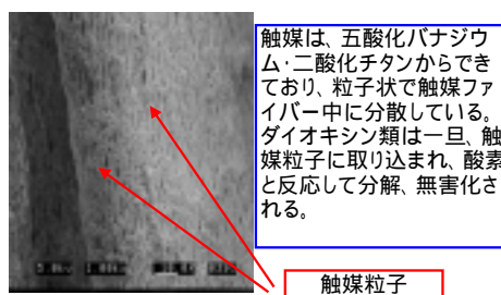
<触媒ファイバー拡大>
