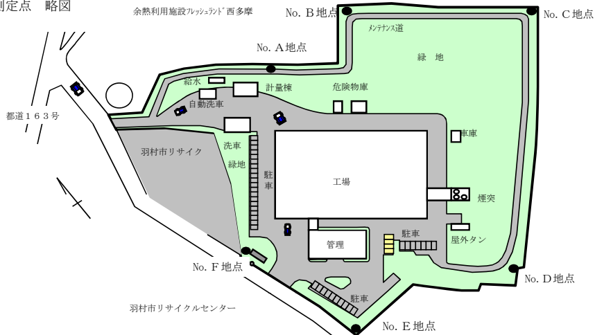
敷地境界線騒音測定点 略図
