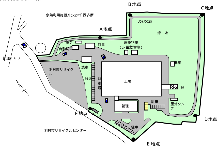
敷地境界線騒音測定点 略図
